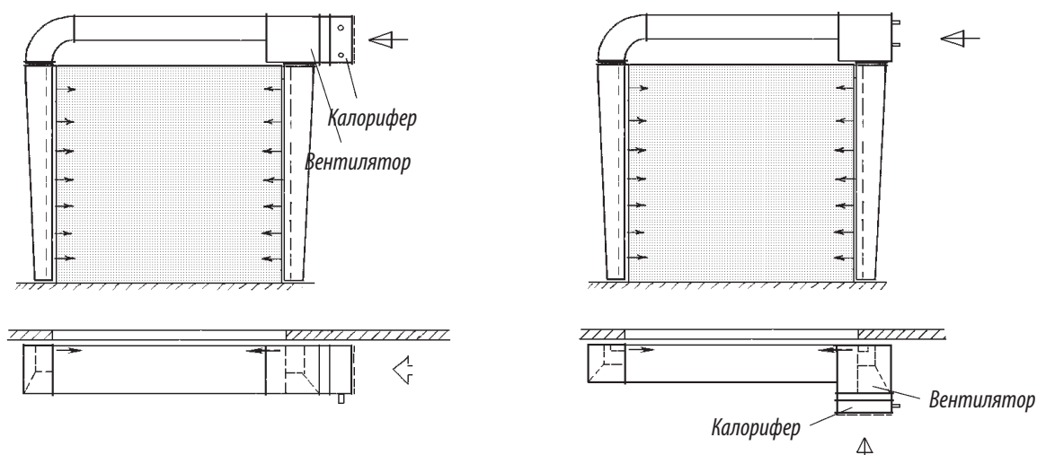
Е. Нагревательный блок в плоскости ворот
