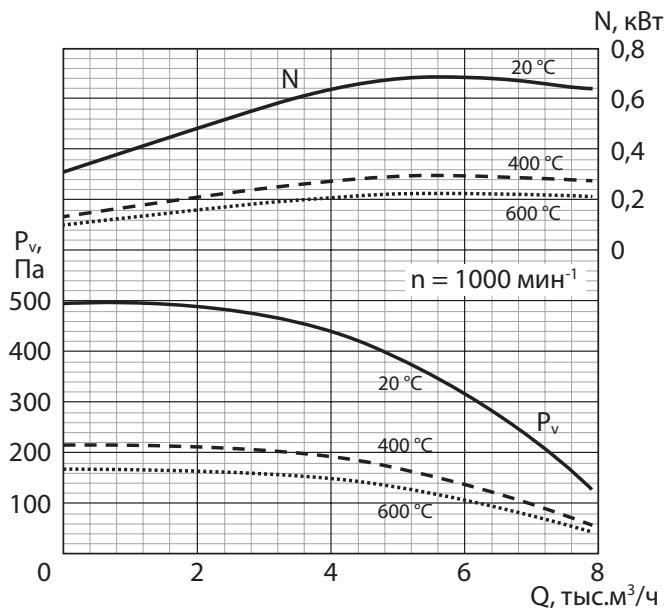
РАДИВЕЙ-ДУ-14-5,6
