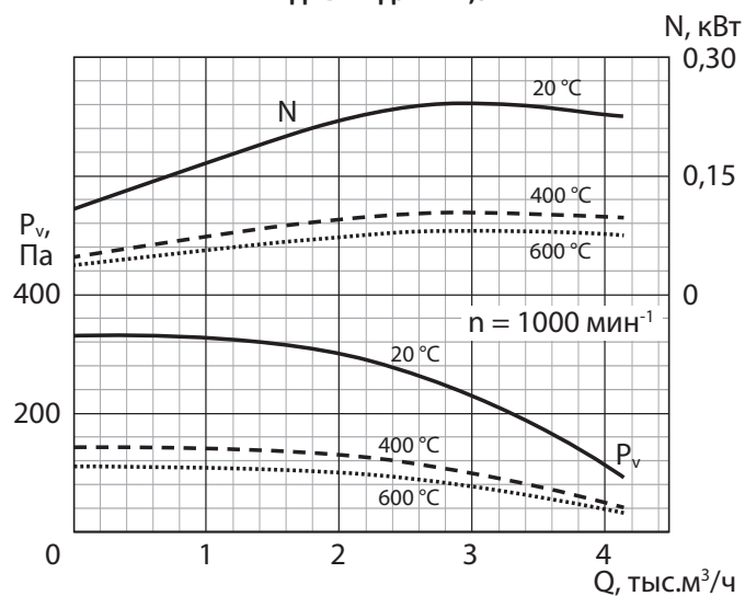
РАДИВЕЙ-ДУ-14-4,5
