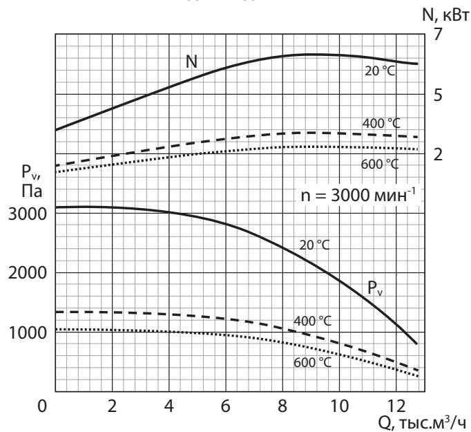
РАДИВЕЙ-ДУ-14-4,5
