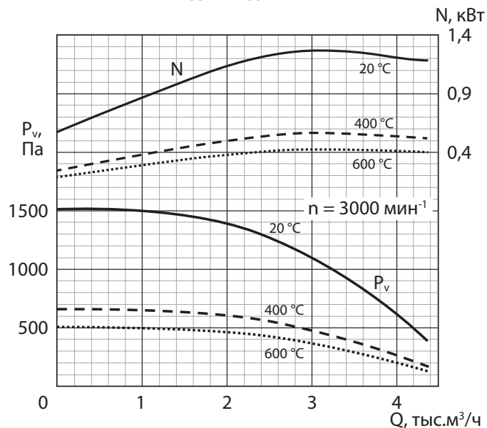
РАДИВЕЙ-ДУ-14-3,15
