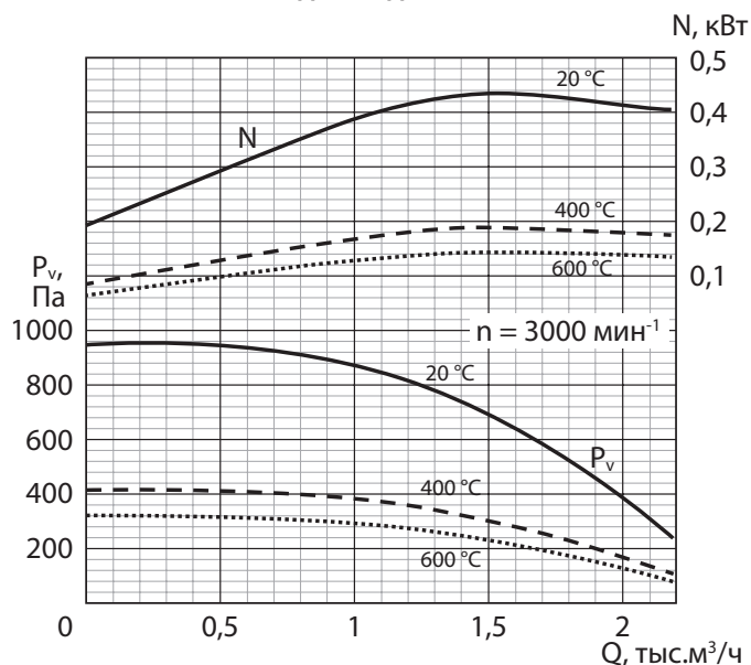
РАДИВЕЙ-ДУ-14-2,5
