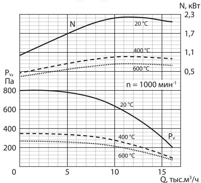
РАДИВЕЙ-ДУ-14-7,1
