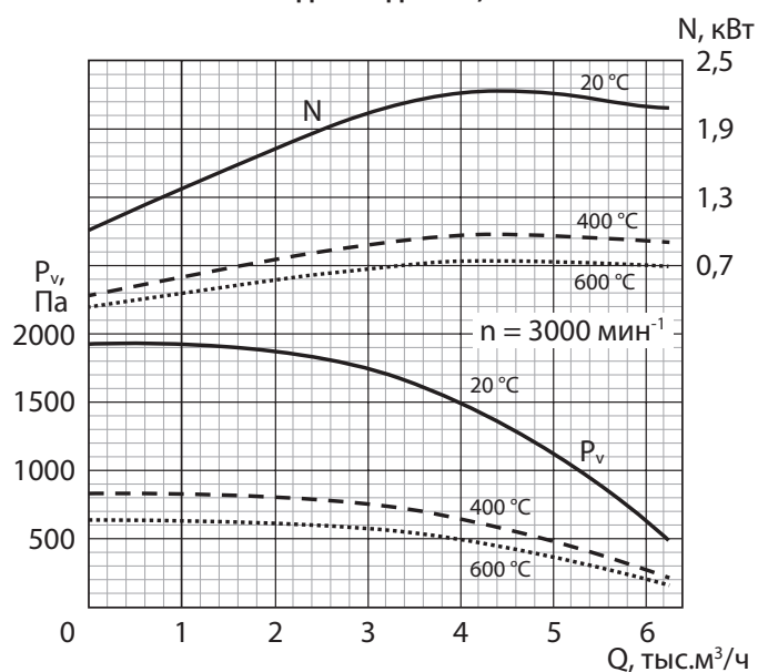
РАДИВЕЙ-ДУ-14-3,55
