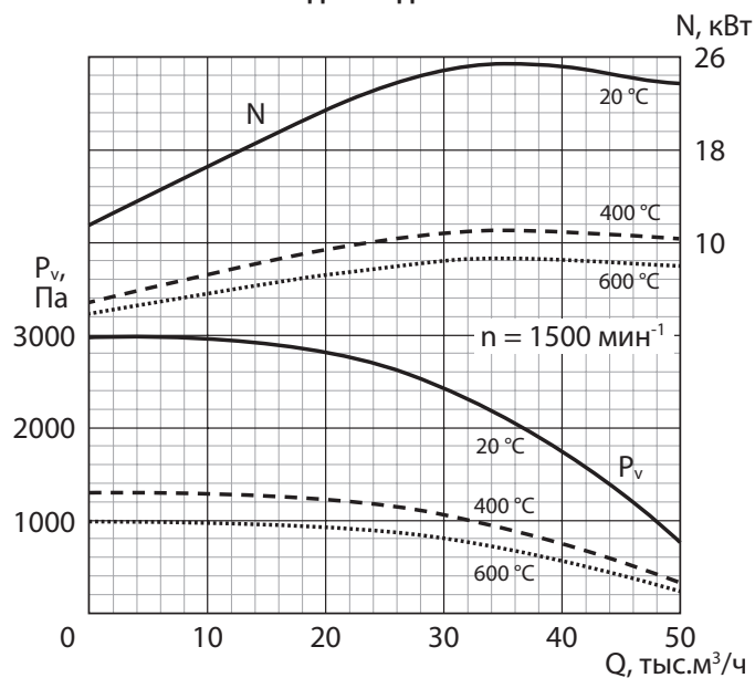
РАДИВЕЙ-ДУ-14-9
