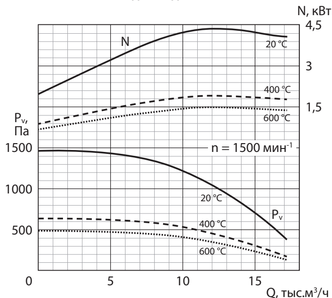
РАДИВЕЙ-ДУ-14-6,3
