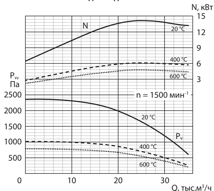
РАДИВЕЙ-ДУ-14-8
