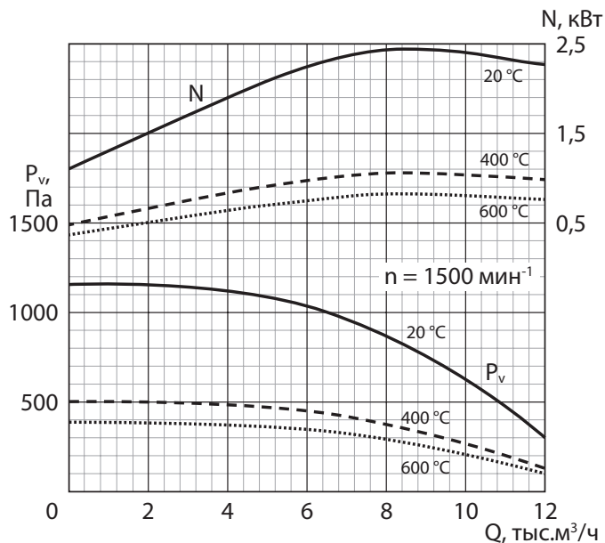
РАДИВЕЙ-ДУ-14-5,6
