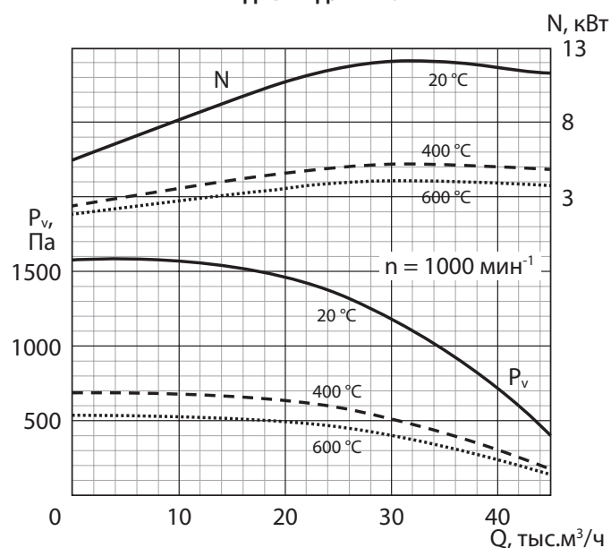
РАДИВЕЙ-ДУ-14-10
