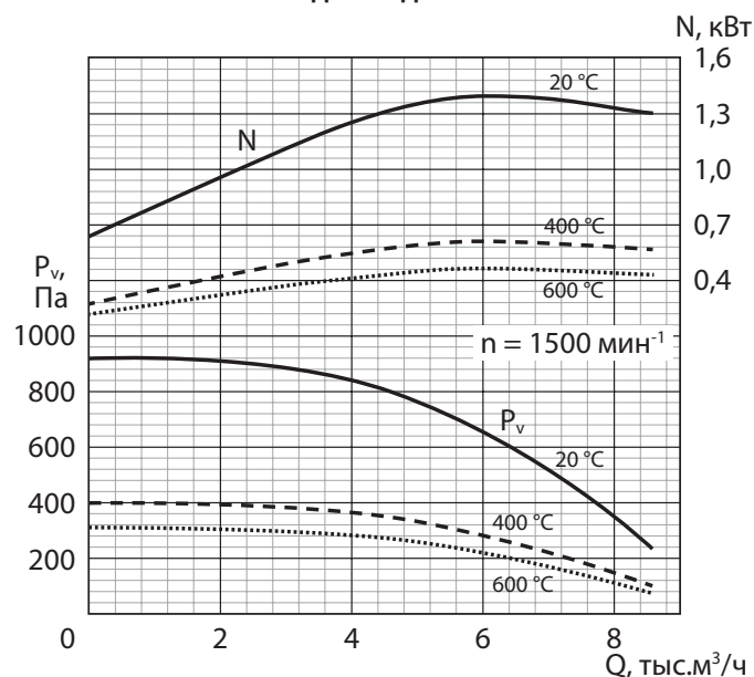
РАДИВЕЙ-ДУ-14-5
