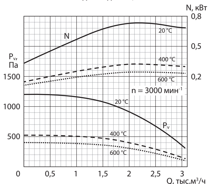
РАДИВЕЙ-ДУ-14-2,8
