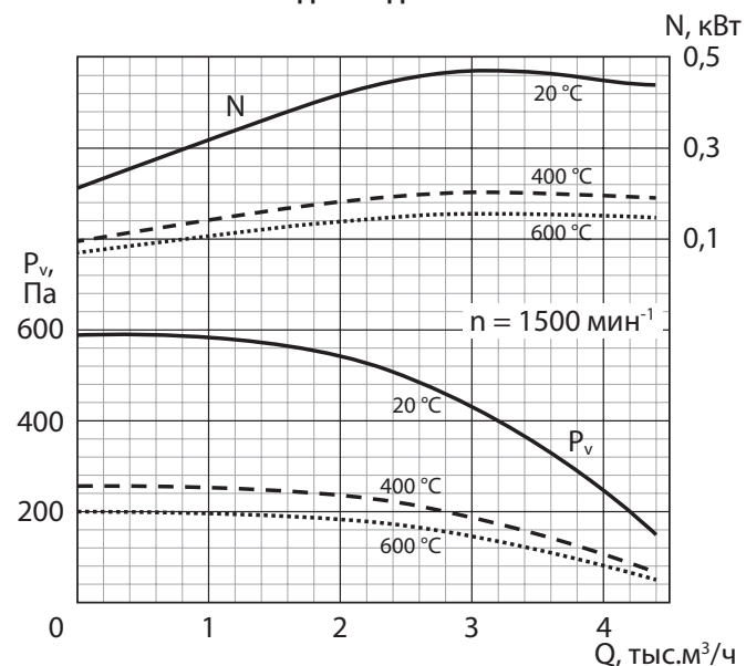
РАДИВЕЙ-ДУ-14-4
